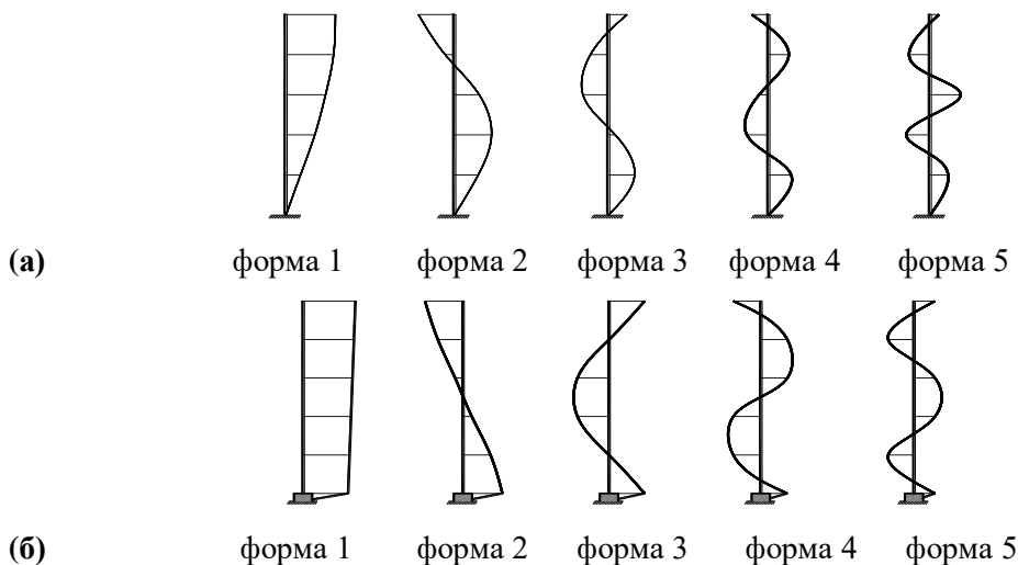
6.2 – сурет – Суперқұрылымның өзіндік көлденең тербелістерінің формалары:
