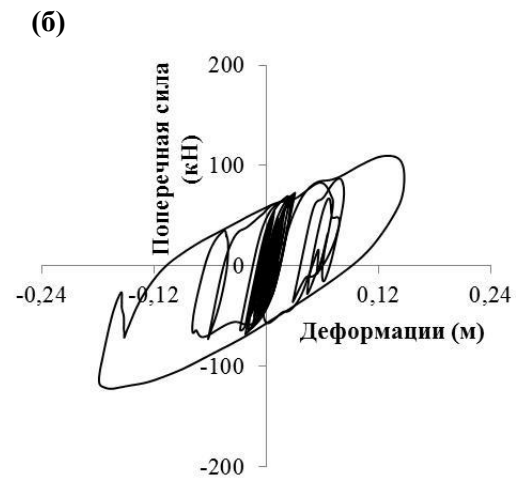
Г2.30-сурет – IZT жасанды акселерограммаларымен берілген "1" сейсмикалық әсерлердің комбинациясы кезінде ғимараттың бойлық (а) және көлденең (б) бағыттарындағы сейсмикалық оқшаулағыш эластомерлік тіректердің әрекетін сипаттайтын тәуелділіктер
