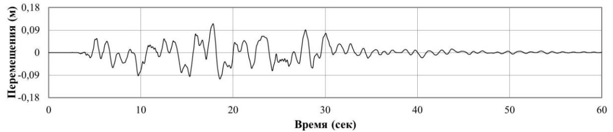
Г2.31-сурет – TCU089 жасанды акселерограммаларымен берілген "1" сейсмикалық әсерлердің комбинациясы кезінде бойлық (а) және көлденең (б) бағыттардағы Суперқұрылым негізінің деңгейінде көлденең үдеу және уақыт бойынша орын ауыстыру
