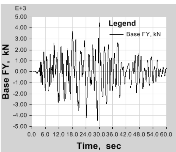
Рисунок Г1.25 – Величины поперечных сил в уровне основания сейсмоизолированной Суперструктуры при комбинации «2» сейсмических воздействий, заданных искусственными акселерограммами А-STU (а), IZT (б) и TCU089 (в)
