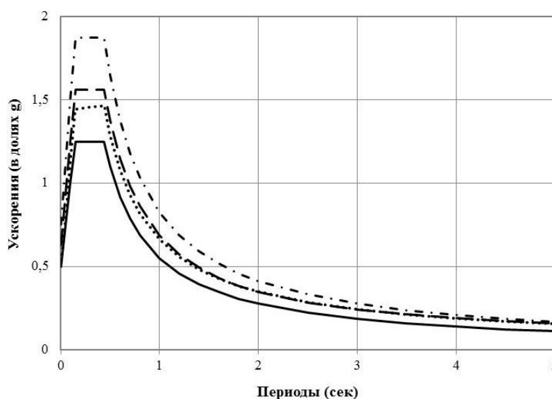
Б.2-сурет – 14 қабатты Суперқұрылымы бар II, III немесе IV жауапкершілік кластарының ғимараттары үшін салынған \xi=5\% кезіндегі серпімді реакциялар спектрлері
