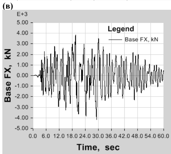
Г2.33-сурет – А-STU (а), IZT (б) және TCU089 (в) жасанды акселерограммаларымен берілген сейсмикалық әсерлердің "1" комбинациясы кезіндегі Суперқұрылым негізінің деңгейіндегі көлденең күштердің шамалары
