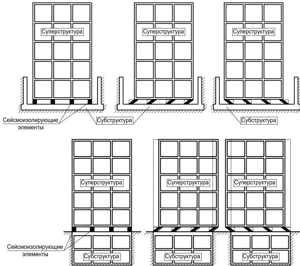
4.1-сурет – Сейсмикалық оқшауланған ғимараттардың көлденең кескіндерінің сұлбалық түрлері
