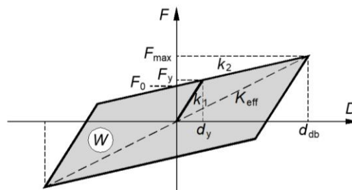
Рисунок 6.3 – Идеализированная зависимость нагрузка-перемещения (F-D), характеризующая поведение сейсмоизолирующей эластомерной опоры с высокой способностью к диссипации энергии и опоры со свинцовыми сердечниками
