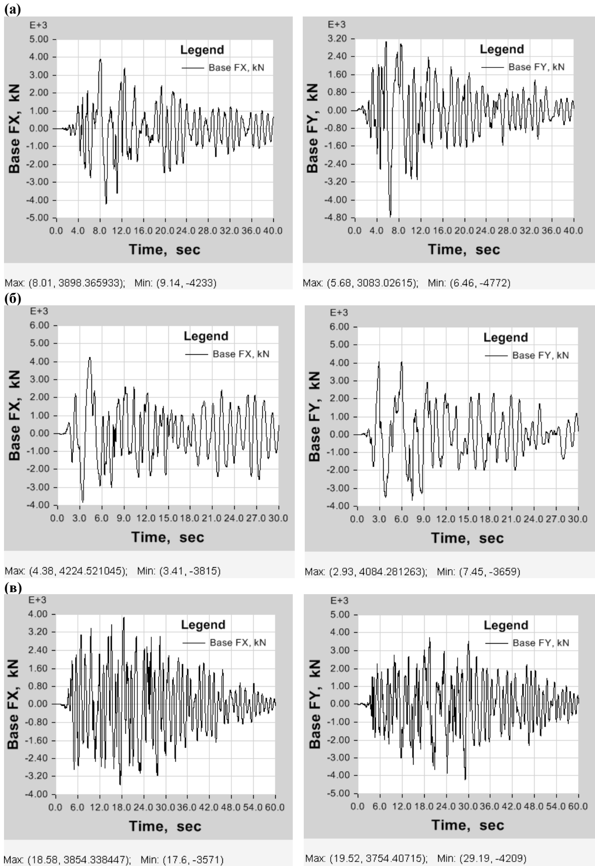
Рисунок Г2.34 – Величины поперечных сил в уровне основания Суперструктуры при комбинации «2» сейсмических воздействий, заданных искусственными акселерограммами A-STU (а), IZT (б) и TCU089 (в)
