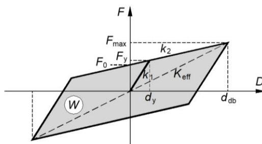
6.3-сурет – Идеалдандырылған жүктеме-орын ауыстыру тәуелділігі (F-D), энергияны диссипациялау қабілеті жоғары сейсмикалық оқшаулағыш эластомерлік тіректің және қорғасын өзектері бар тіректің беталысын сипаттайды
