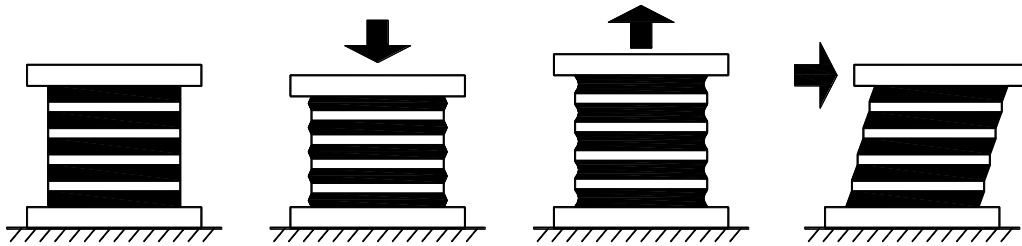
2.4 - сурет – Тік және көлденең жүктемелер кезінде эластомерлік тіректердің деформациясы
