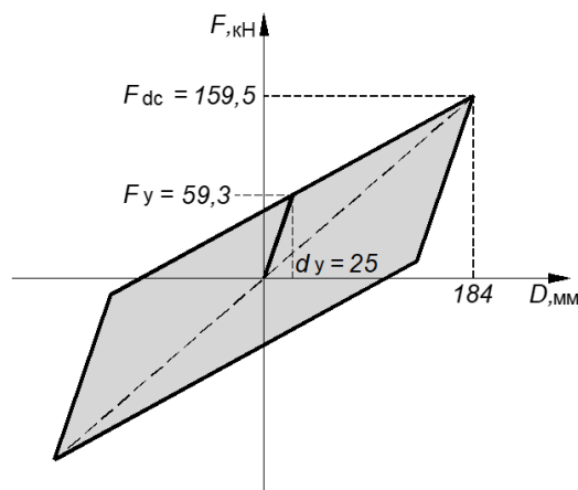
В.2-сурет – Энергия диссипациясының жоғары қабілеті бар сейсмикалық оқшаулағыш эластомерлік тіректің беталысын сипаттайтын жүктеме-орын ауыстырудың идеалдандырылған тәуелділігі ( F-D ), В (1)-мысалында қарастырылған
