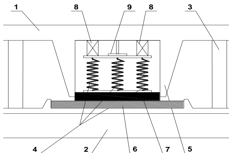
Рисунок Е.2 - Демпферы сухого трения:
